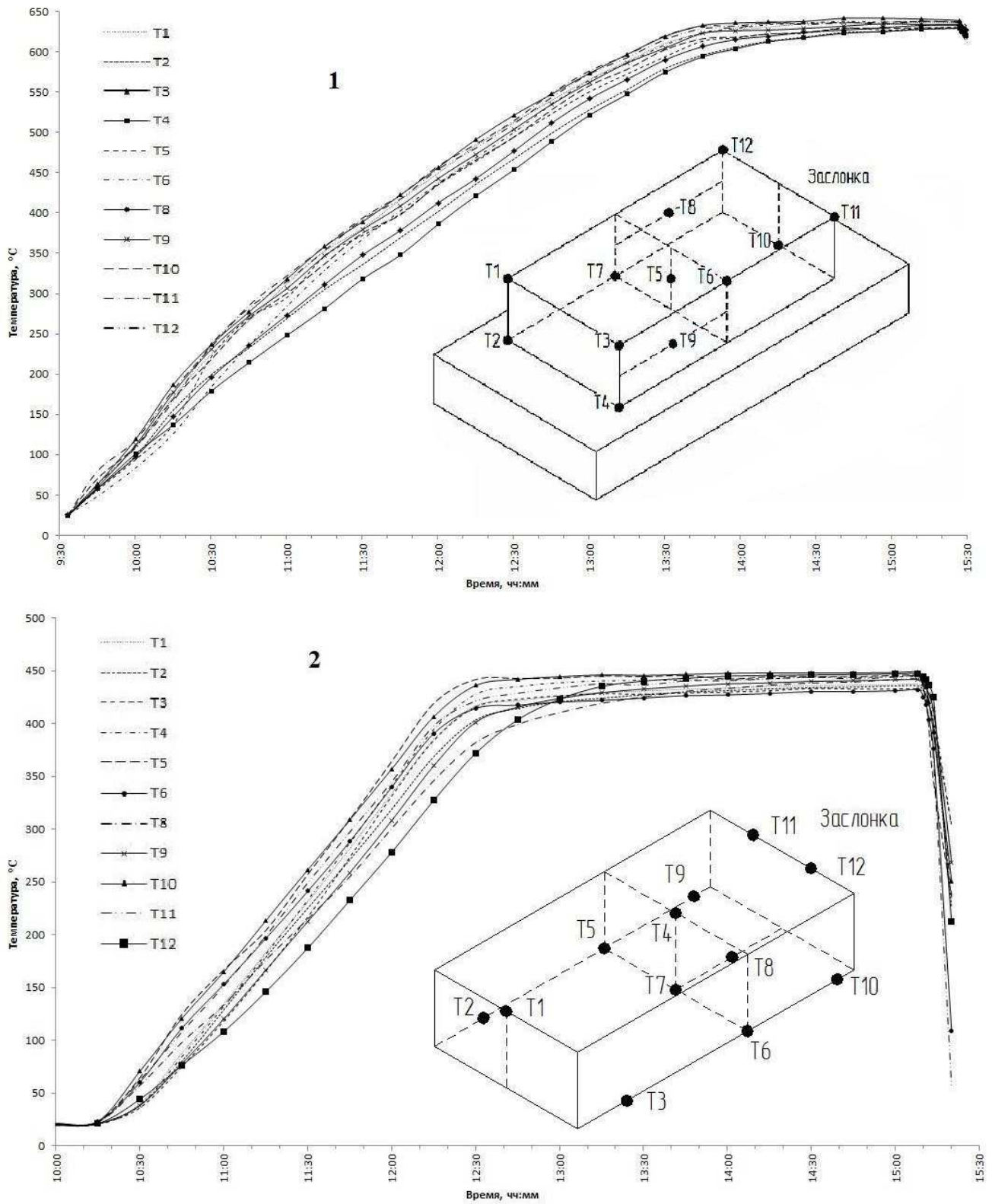
Рис.5. Термограмма нагрева специзделий: 1-специзделие №1, 2-специзделие №2
