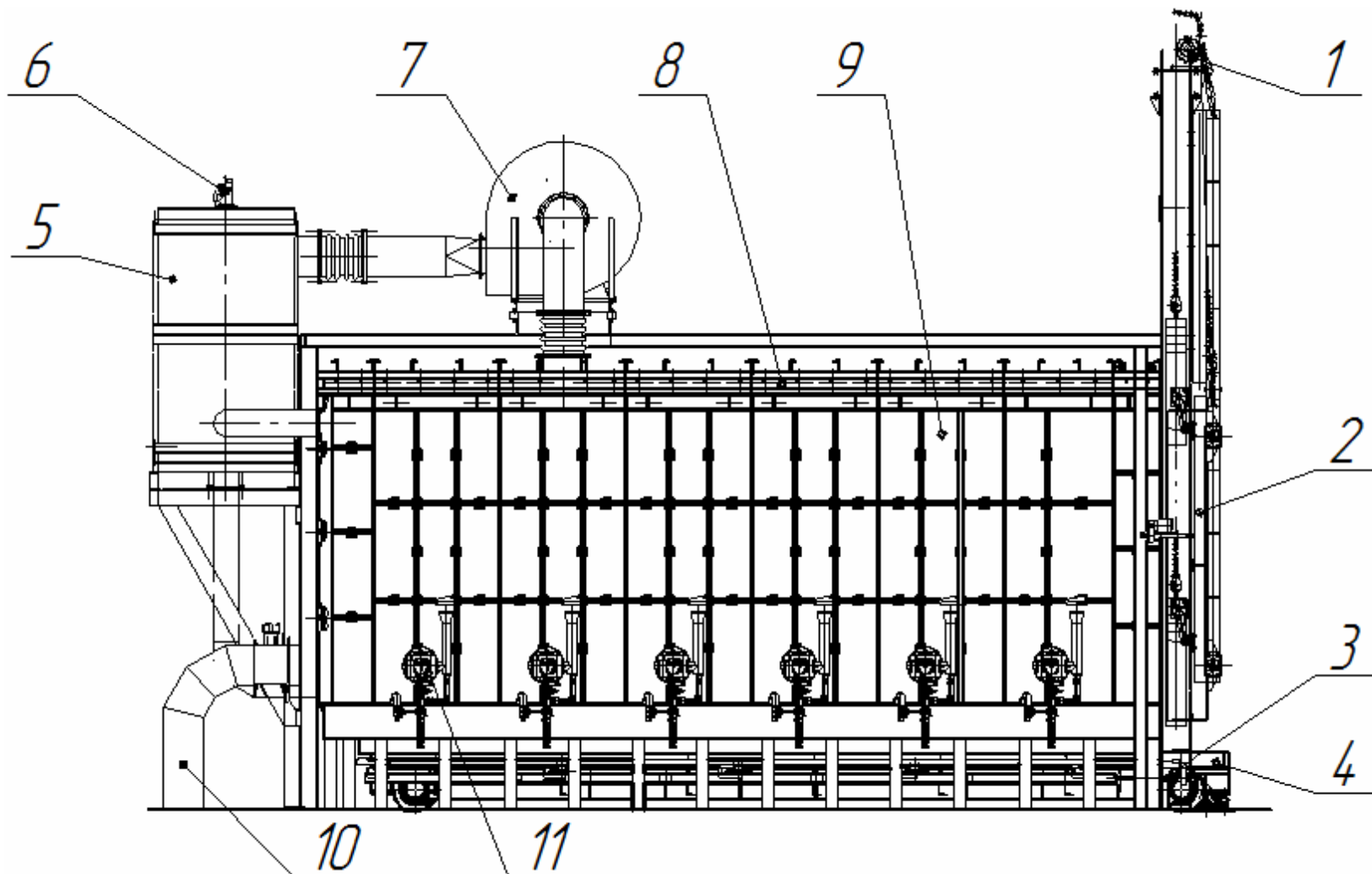
Рис. 1. Эскиз печи, боковой вид: 1 – механизм подъема заслонки; 2 – подвижные направляющие механизма прижима заслонки; 3 – привод механизма уплотнения пода; 4 – выкатной под; 5 – камера подогрева рециркулята; 6 – горелка камеры подогрева рециркулята; 7 – рециркуляционный вентилятор; 8 – сводовые панели; 9 – боковые панели; 10 – дымоотводящий канал; 11 – основные горелки
