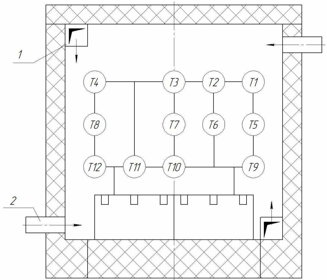
Рис.2. Схема размещения термопреобразователей на раме передвижной:
